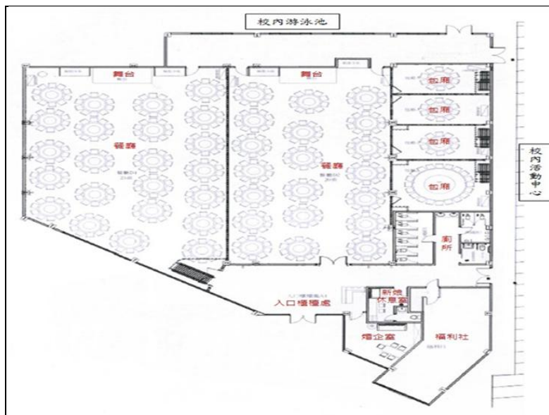
斗六家商實習商店 BOT 契約變更後平面配置圖
